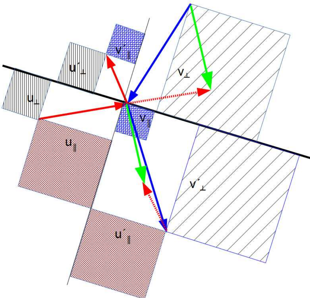
Abbildung 4: Impuls- und Energieerhaltung (schwarz Stoßachse und auf Atom erhaltene Komponenten, rot u' 's blau v' 's, grün erhaltene Relativgeschwindigkeit => Impuls)
