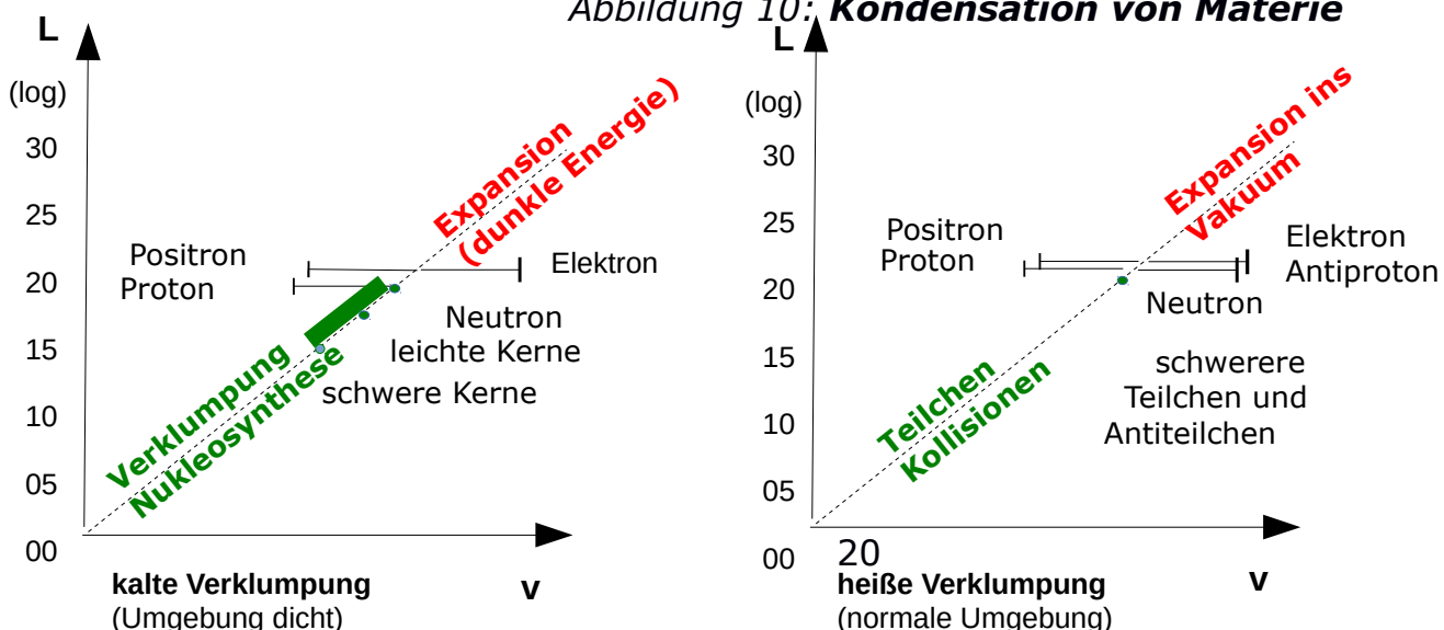
Abbildung 10: Kondensation von Materie
